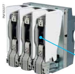
Контактная площадка без дефлектора
